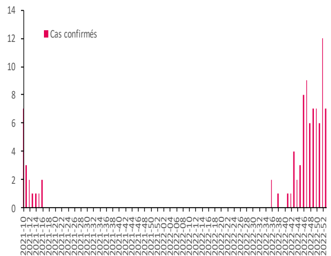
Figure 1 : Nombre hebdomadaire de cas biologiquement confirmés par NS1 et/ou RT-PCR, Guadeloupe, semaines 2021-10 à 2023-01. Source : Laboratoires de ville, CNR, CHU, CHBT IP Guadeloupe, Cerba, Biomnis.
